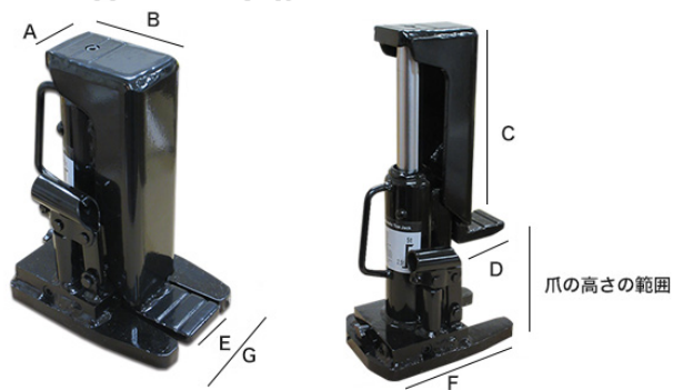
各部分の寸法（単位：mm）
